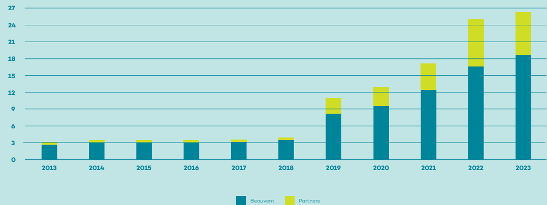
Vermogen zonne-installaties Beauvent (MWp)
